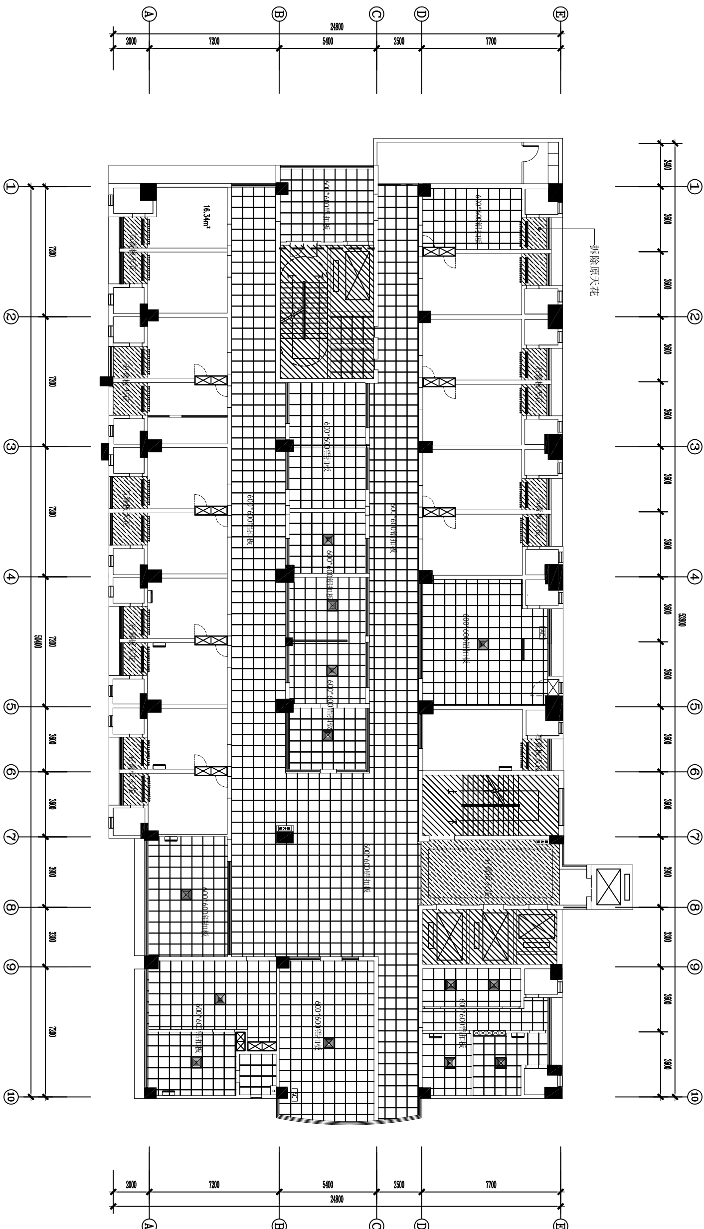
ARCHITECTURAL INFO. PLAN 人医住院楼三楼普外科拆除原天花平面图 SCALE 1:200
