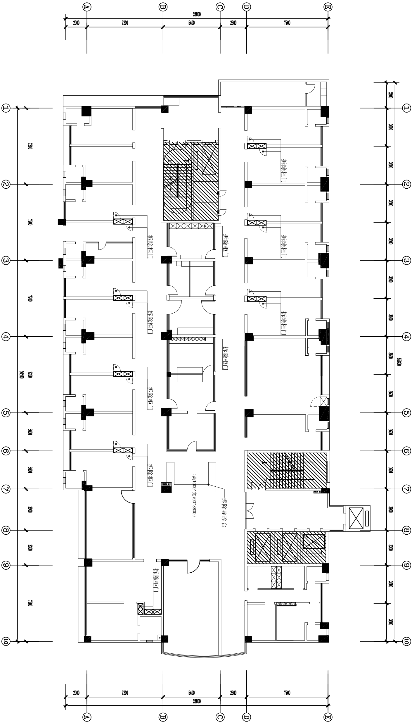
ARCHITECTURAL INFO. PLAN 人医住院楼三楼普外科更换柜门平面图 SCALE 1: 200
