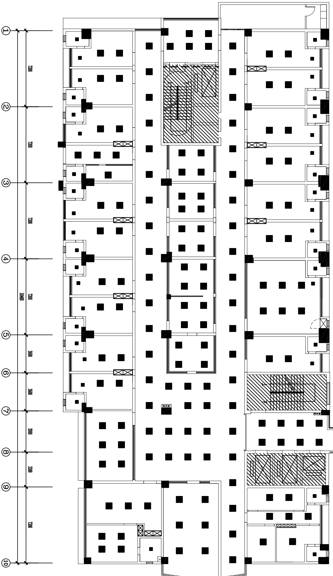
ARCHITECTURAL INFO. PLAN 人医住院楼三楼普外科照明平面图 SCALE 1:200
