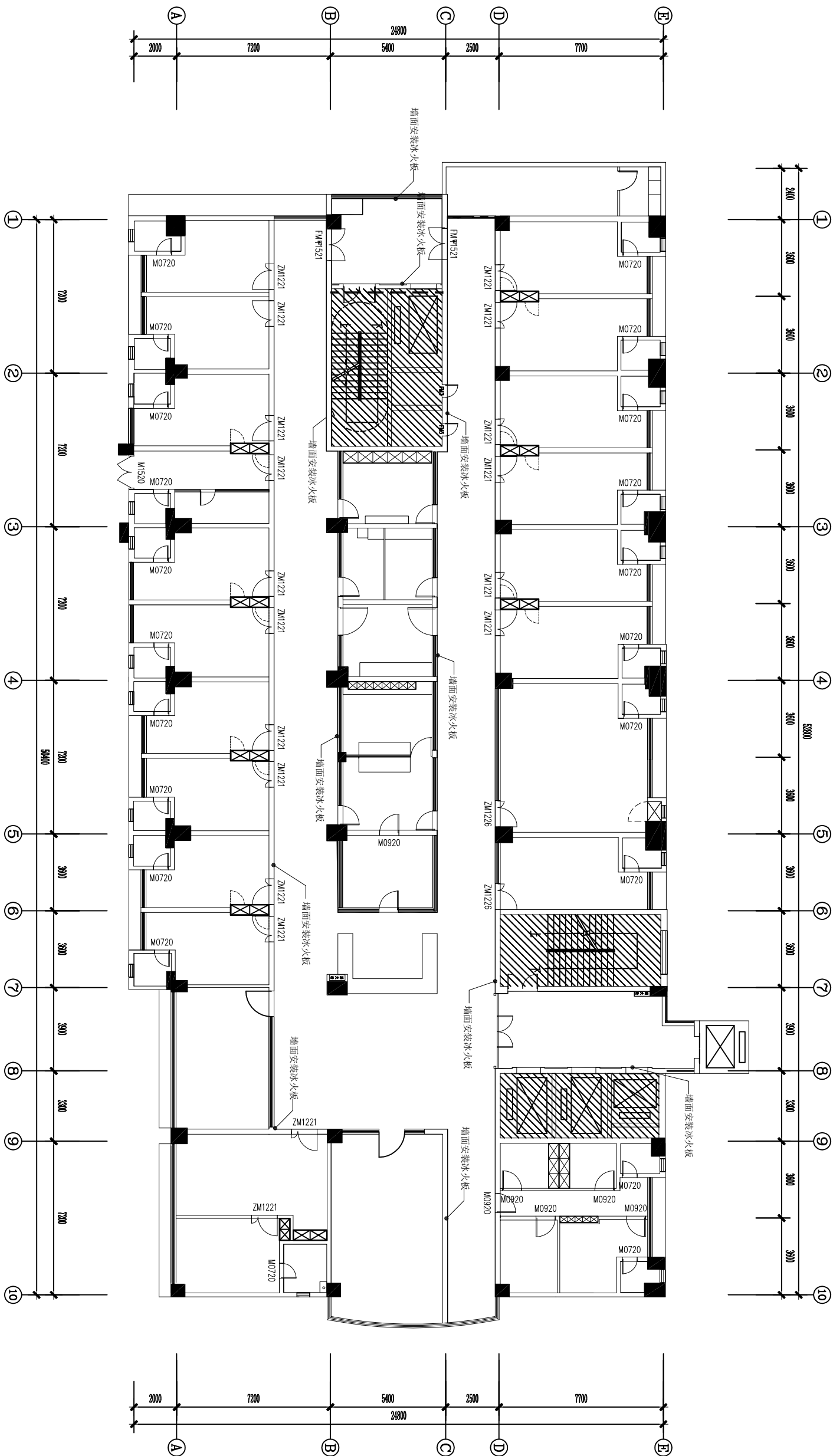
ARCHITECTURAL INFO PLAN 人医住院楼三楼普通墙面安装冰火板平面图 SCALE 1: 200
