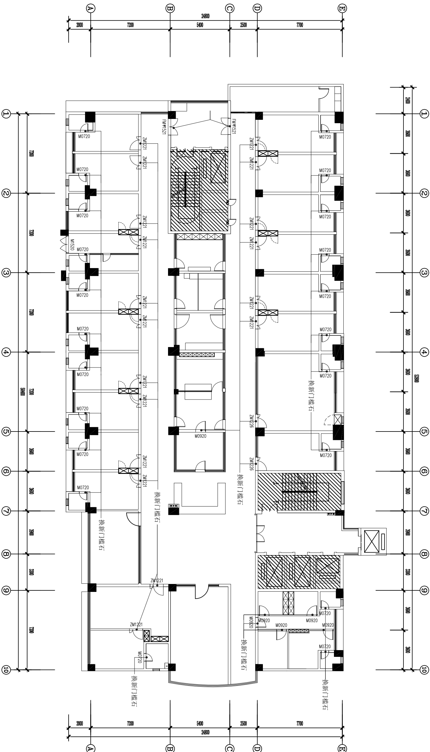
ARCHITECTURAL INFO. PLAN 人医住院楼三楼普外科门槛石换新平面图 SCALE 1:200
